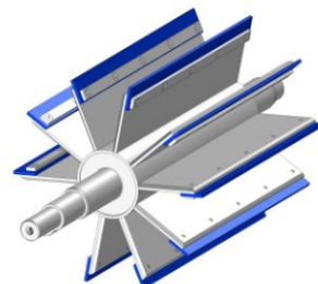
Мягкие 3-сторонние лопасти
