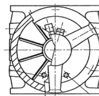
Отверстие продувания ячеек
