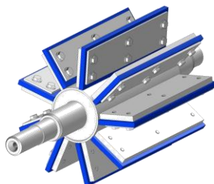
Мягкие 1-сторонние лопасти
