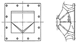
Дефлектор с защитой от усилия сдвига
