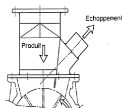
Деаэрационная коробка
