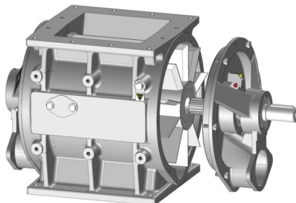
Боковой проход - Side passage
